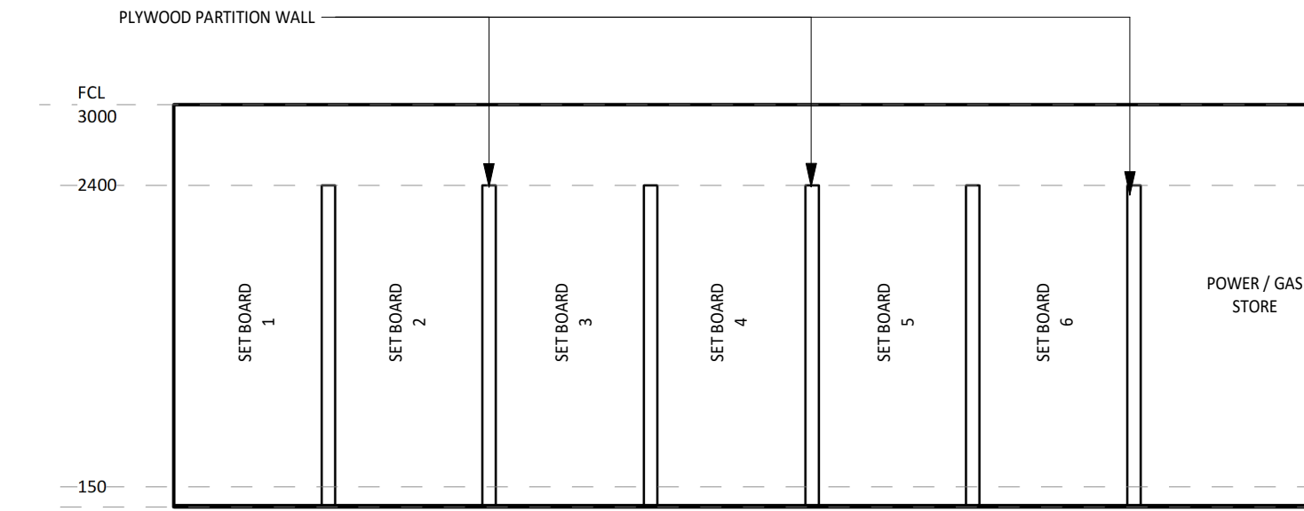
5 ELEVATION DETAIL 60-042 1 : 50
