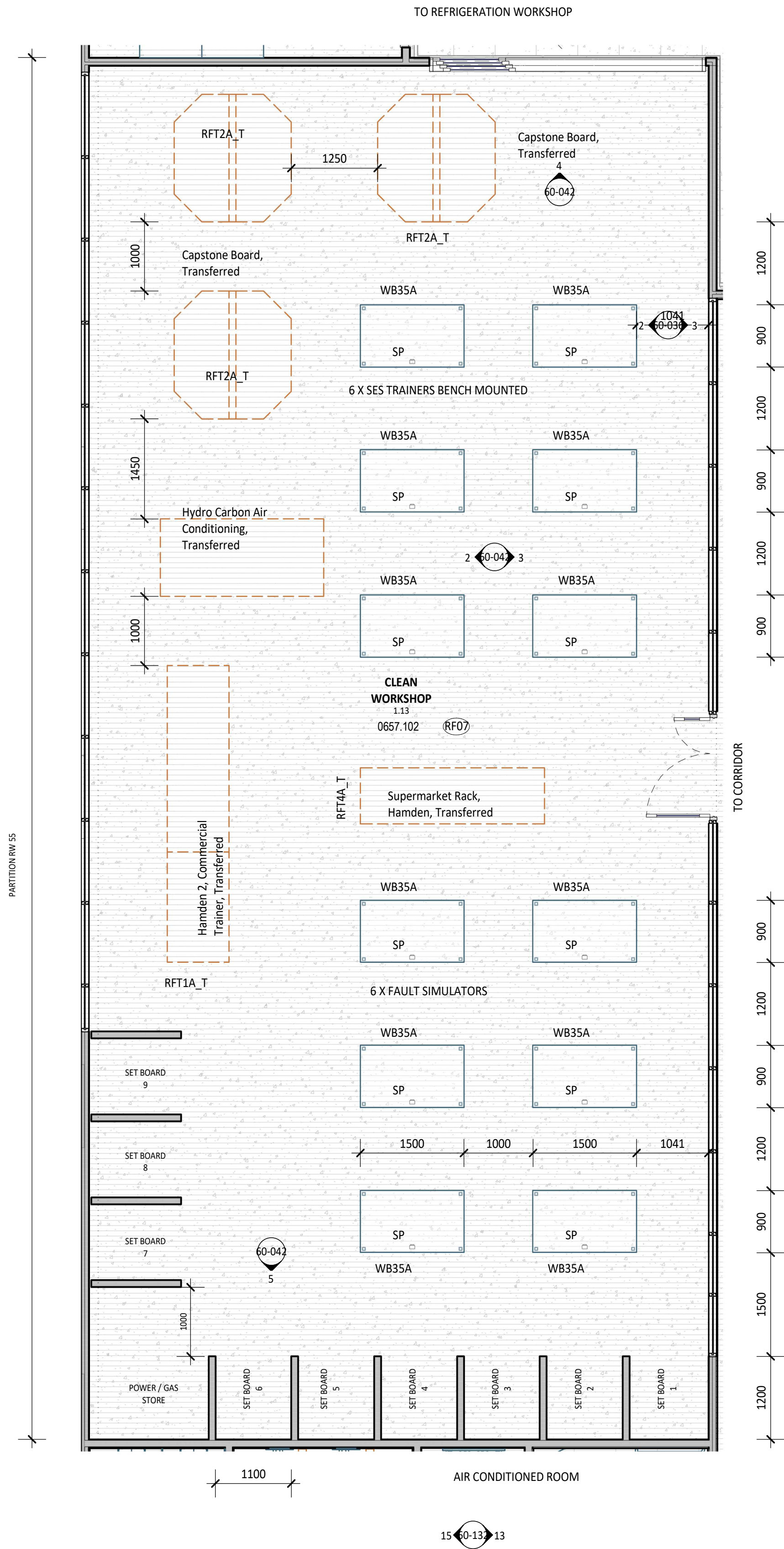
1 PLAN DETAIL 1 : 50
