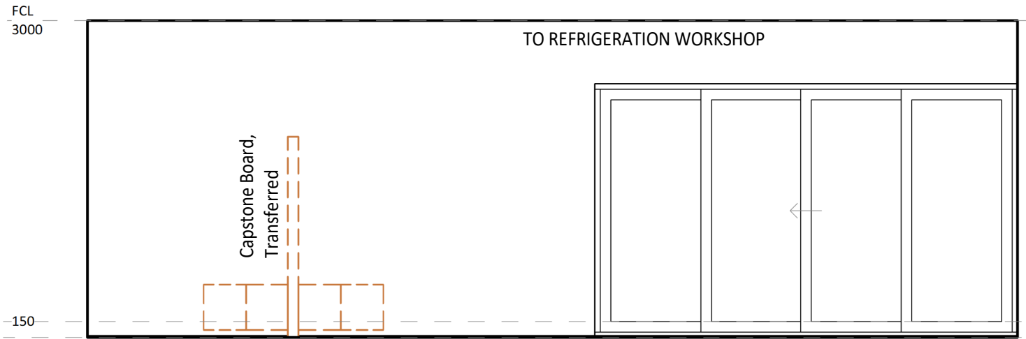
4 ELEVATION DETAIL 60-042 1 : 50
